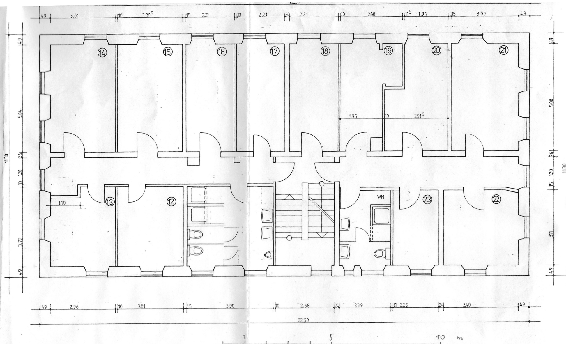
1. OBERGESCHOSS
